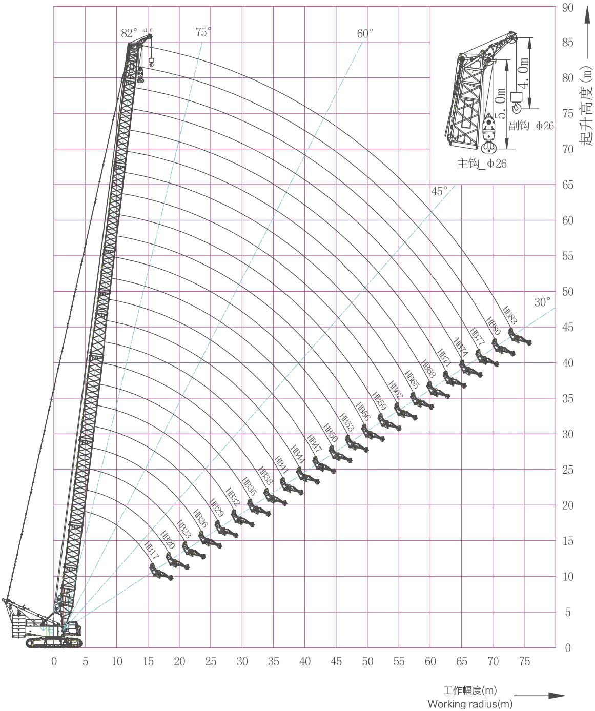
主臂工况_带臂端滑轮(HBS/1)的主臂主钩工作范围图
